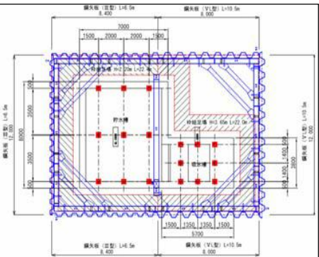
図-1 平面図
