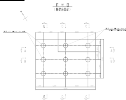
図-1 基礎杭図
