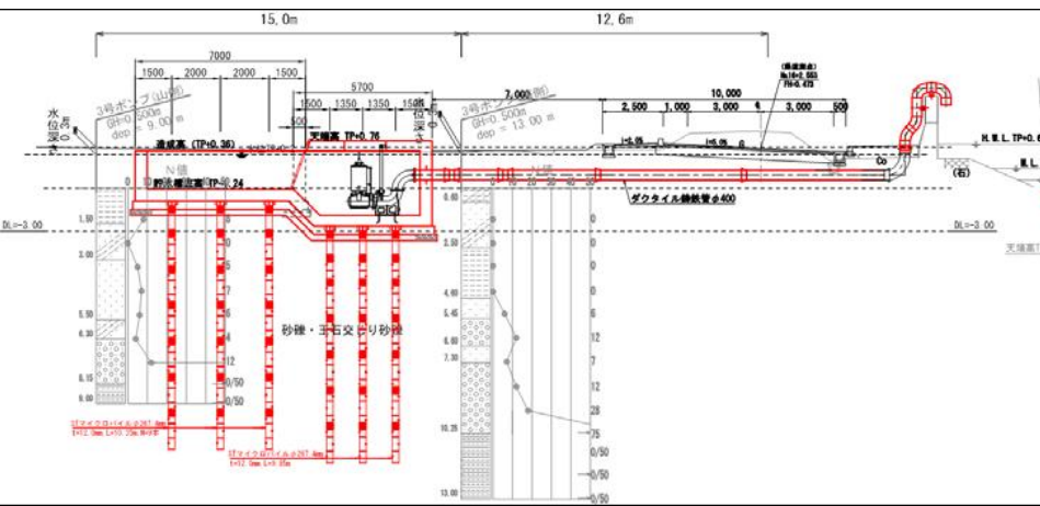
図-2 断面図
