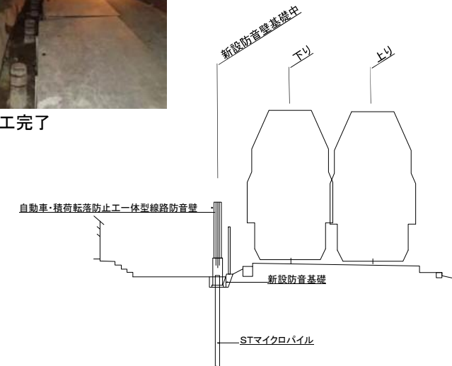
施工概略
