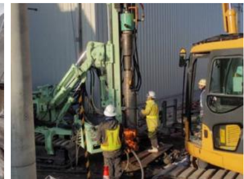
二重管削孔 ( \phi 315.8\text{mm} )
