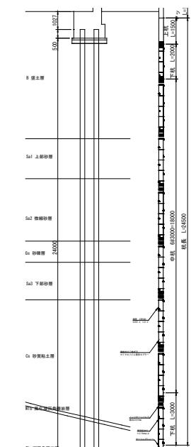
A2橋台
