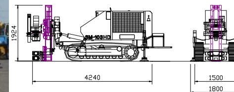
超低空仕様削孔機外觀図
