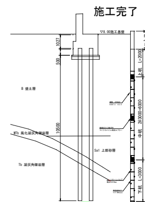
A1橋台
