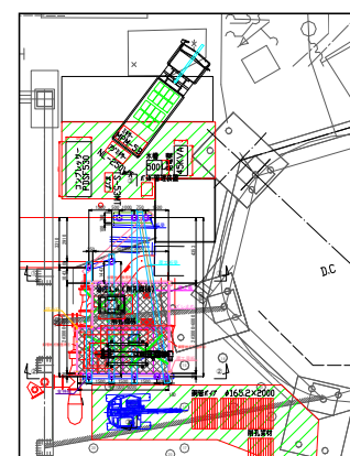
施工状況図
