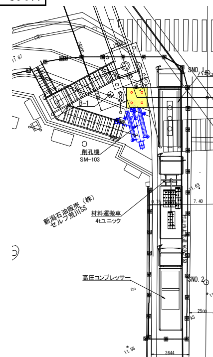
施工平面図
