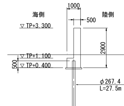
図-1 防潮堤断面図
