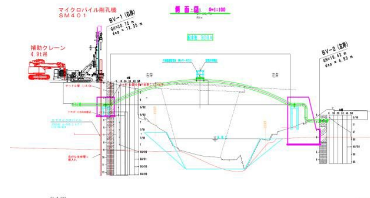
施工状況図
