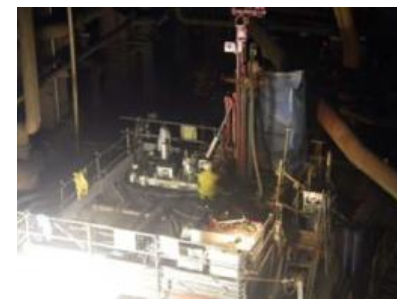
削孔状況
