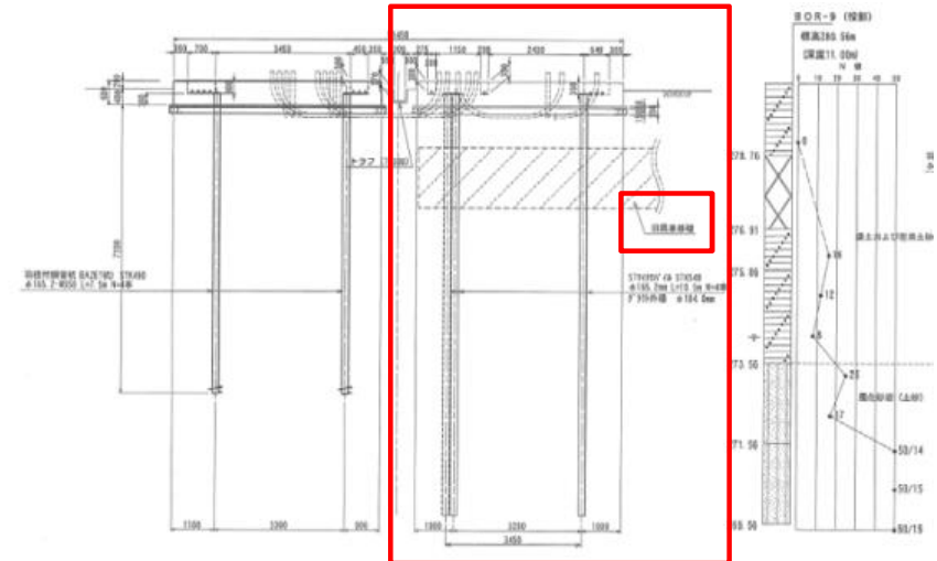
基礎断面図
