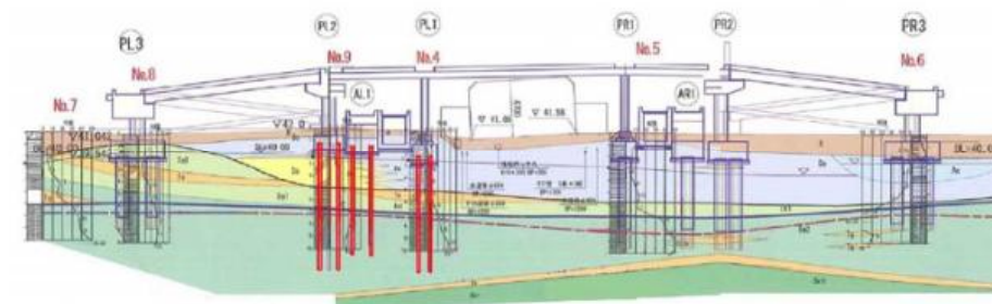
横断歩道橋側面図
