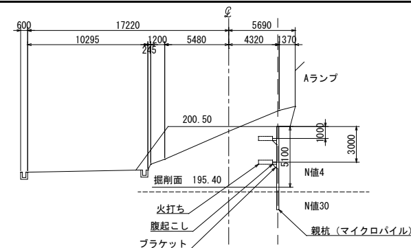
図-1 土留め断面図
