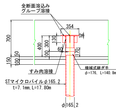
杭頭部詳細図
