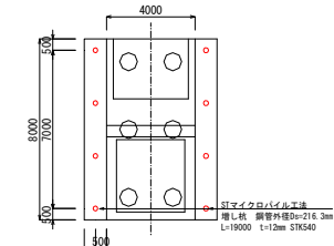
A2橋台 平面図
