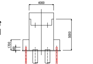
A2橋台 正面図
