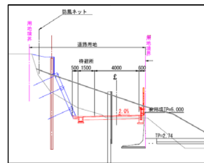
標準断面図
