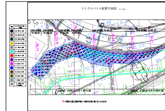
施工平面図
