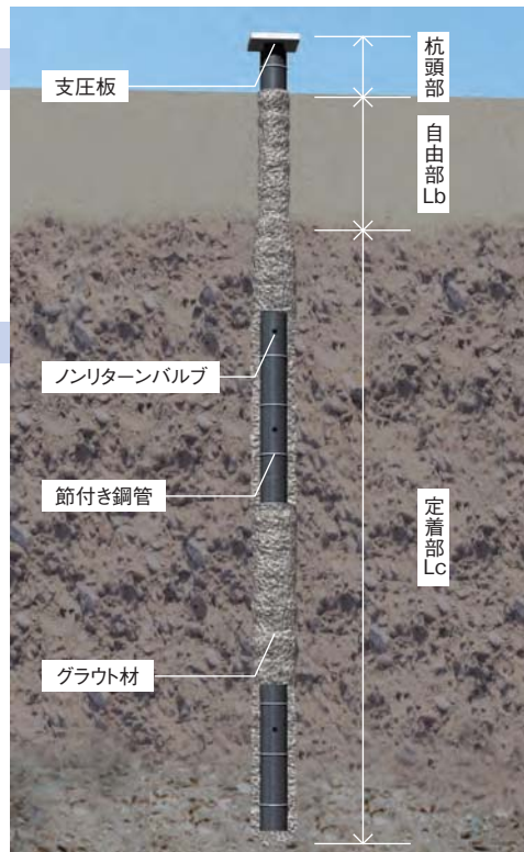
STマイクロパイル工法 タイプⅠ
