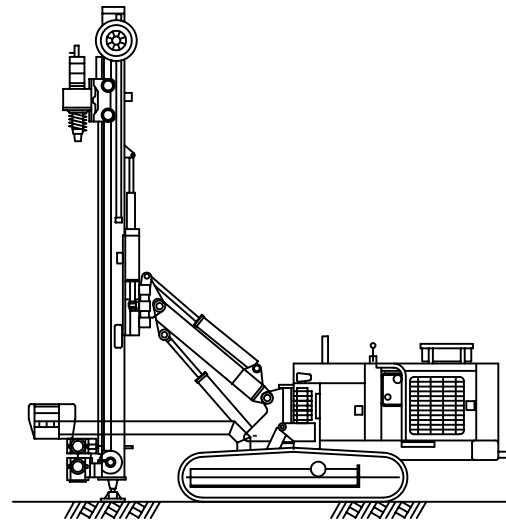
ベースマシン (SM-400の場合)
