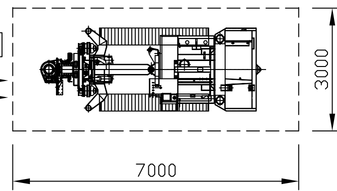
ベースマシン (SM-400の場合)
